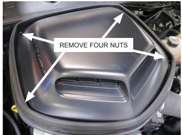
Fig. 2-n: Remove shaker scoop
